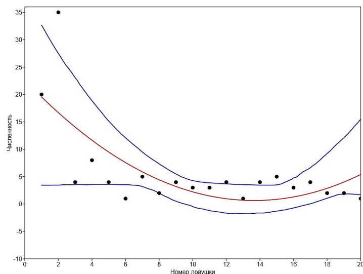
Рисунок 2 – Колебания численности жужелиц по мере удаленности от края зоны отчуждения нефтескважины № 53 Северо-Домановичского нефтяного месторождения
