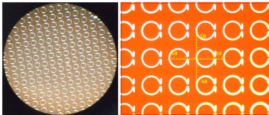
Рисунок 6 – Метаматериал, образованный проводящими омега-элементами на кремниевой подложке (ОАО «ИНТЕГРАЛ», ИФ НАН Беларуси и ГГУ)
