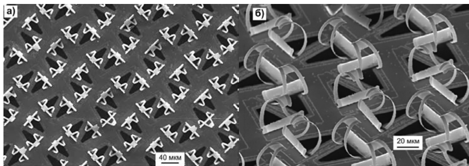
Рисунок 5 – «Невидимый» поглощающий метаматериал для терагерцовой области спектра (Институт физики полупроводников СО РАН, Новосибирск и ГГУ)
